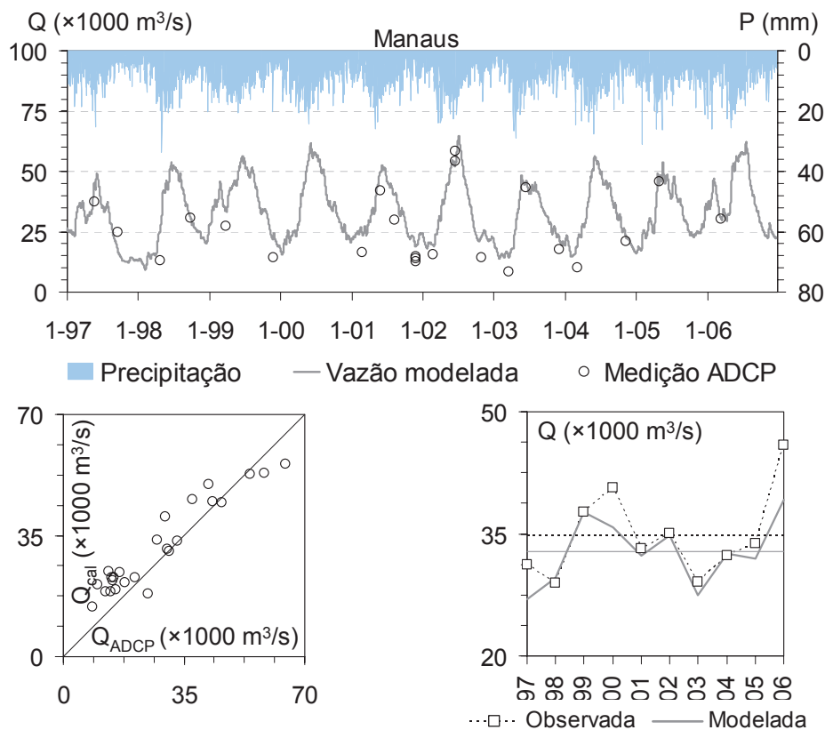
Figura 6 – Resultados do modelo em Manaus: acima, vazões diárias simuladas (linha cinza) e adquiridas por ADCP (círculos); abaixo, à esquerda, gráfico de dispersão das vazões ADCP e simuladas; e, abaixo, à direita, séries de vazões anuais médias simuladas (linha cinza) e observadas (linha pontilhada).
