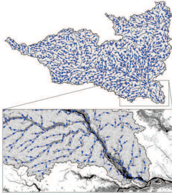
Figura 2 - Representação computacional da bacia do rio Negro. Linhas brancas delimitam mini-bacias. Canais (vetores azuis) conectam os centróides de mini-bacias indicando as direções para o cálculo da propagação. Abaixo, um detalhe da confluência dos rios Negro e Solimões.
