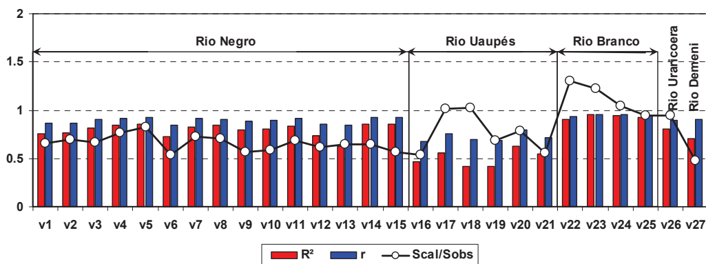
Figura 7 – Resultados obtidos nas 27 estações virtuais consideradas para a etapa de validação dos parâmetros: coeficiente de correlação (r) e determinação ( R^2 ); e razões s_{\text{obs}}/s_{\text{cal}} para avaliar séries temporais de profundidades do rio contra a altimetria espacial obtida pelo satélite ENVISAT.
